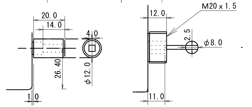
スクエアキータイプ接続部
