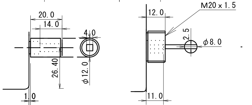
スクウェアキータイプ接続部
