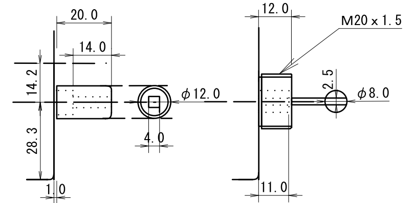
スクウェアキータイプ接続部 フレキシブルシャフトタイプ接続部
