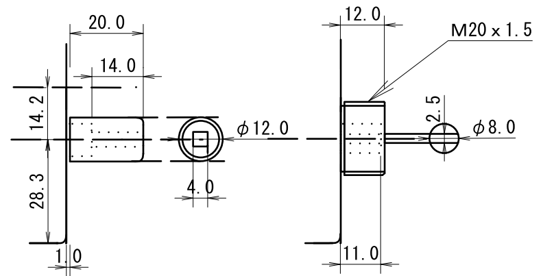
スクウェアキータイプ接続部
